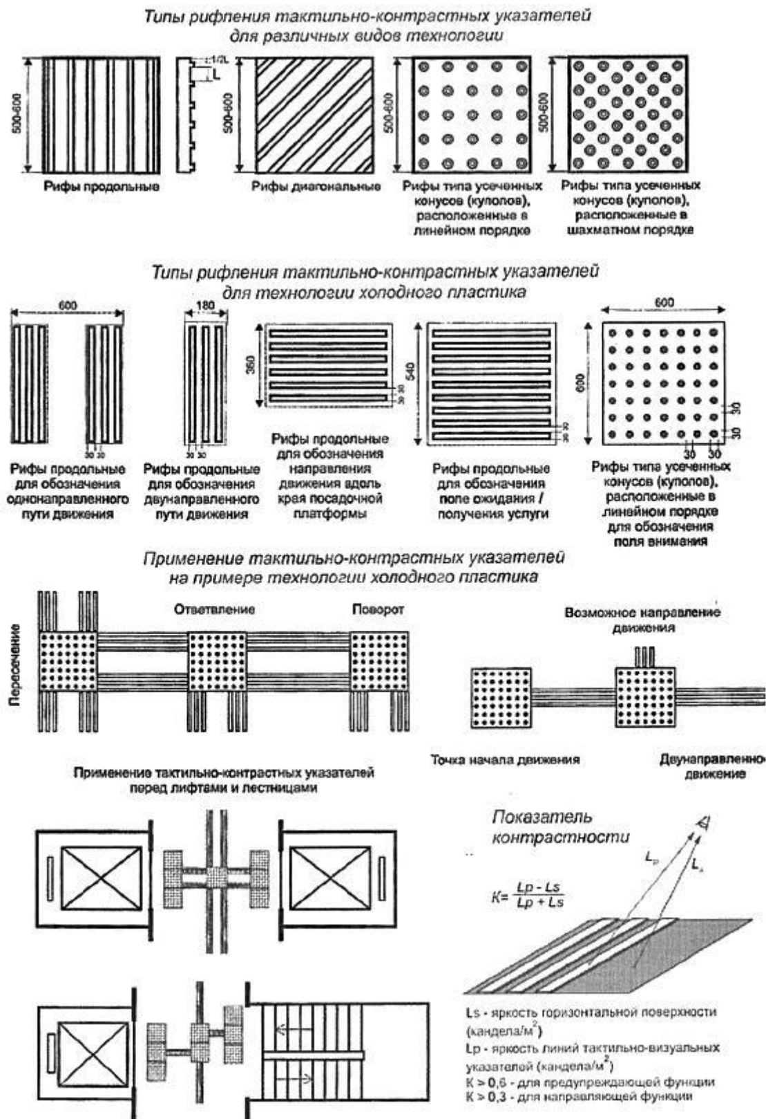
Рисунок Г.18 - Тактильно-контрастные указатели
