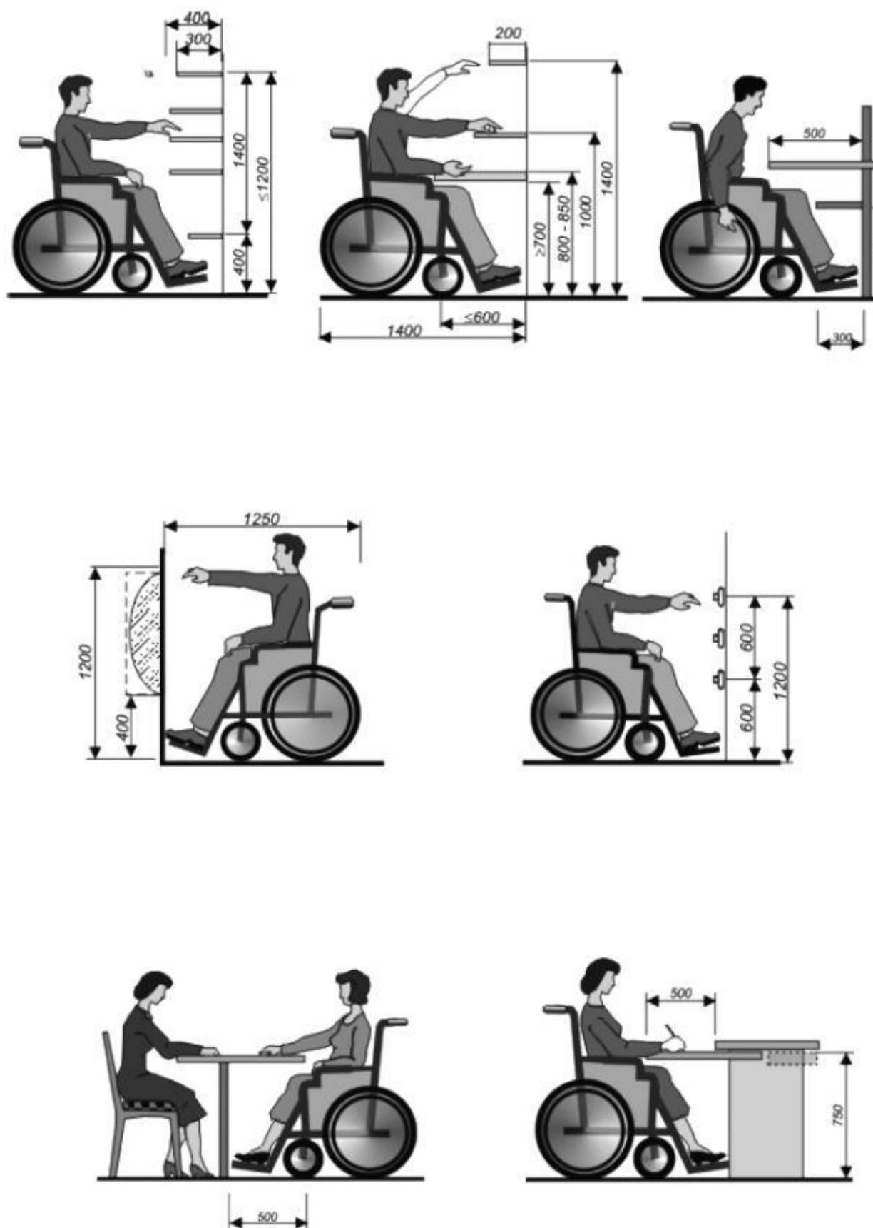
Рисунок Г.2 - Параметры досягаемости в месте получения услуги
