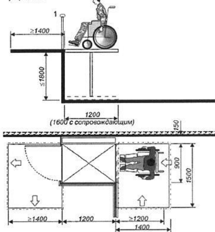
Въездное подъемное устройство
