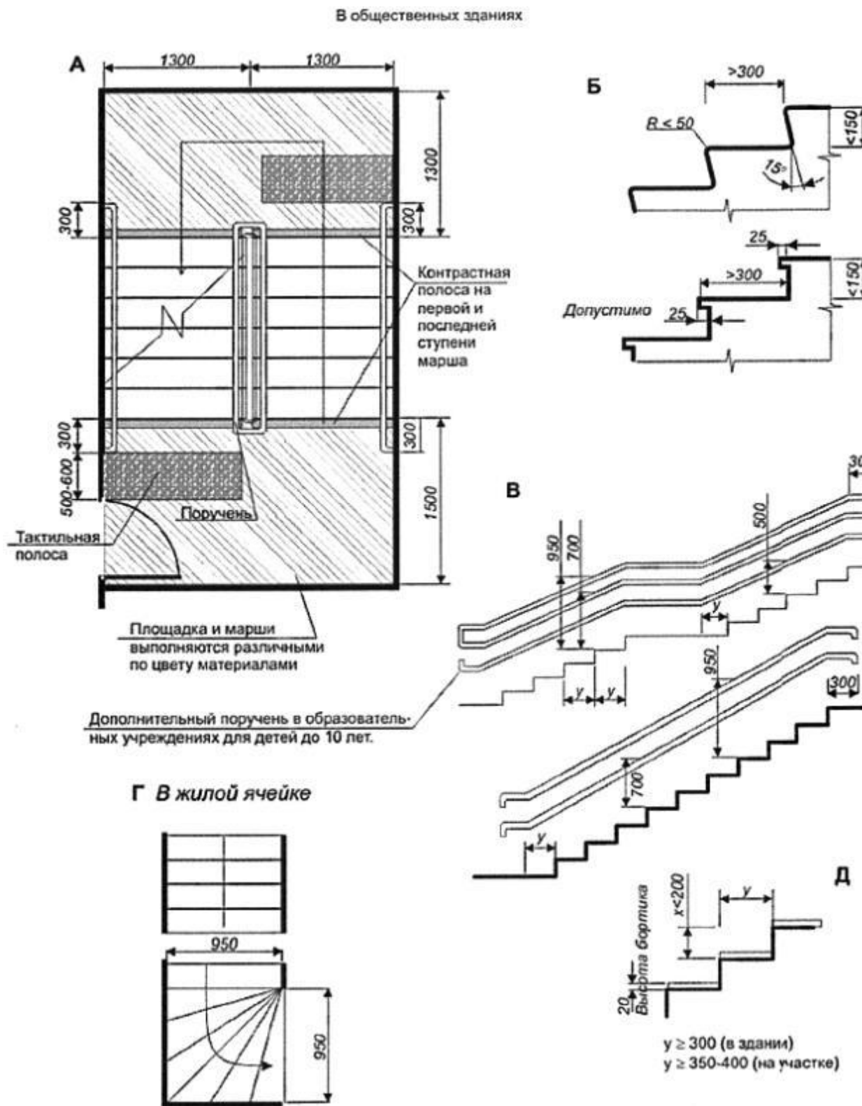
Рисунок В.23 - Лестницы в общественных зданиях и жилой ячейке
