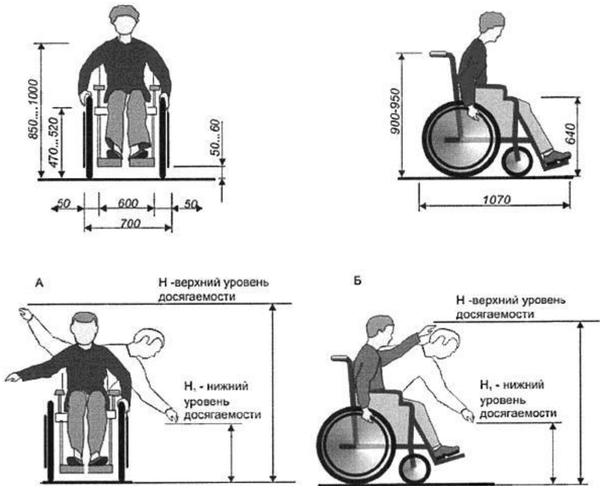
А - при боковом доступе
