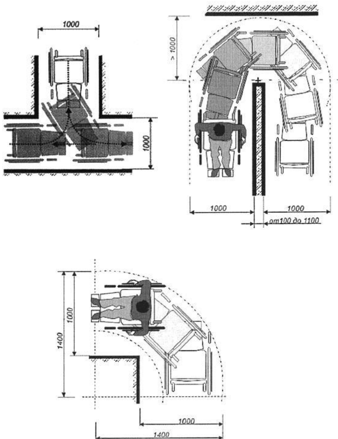
Рисунок В.13 - Размеры поворота и разворота кресла-коляски
