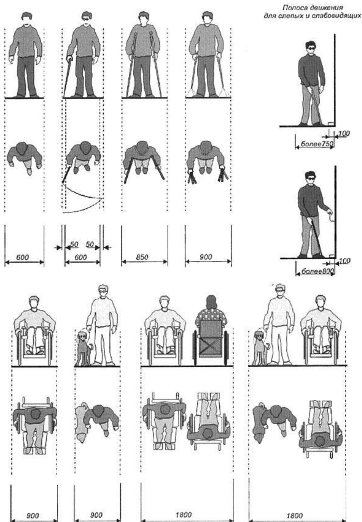
Рисунок В.11 - Габариты
