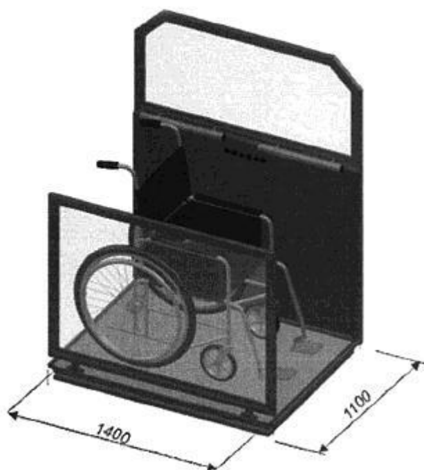
Шахтный подъемник с закрытой платформой
