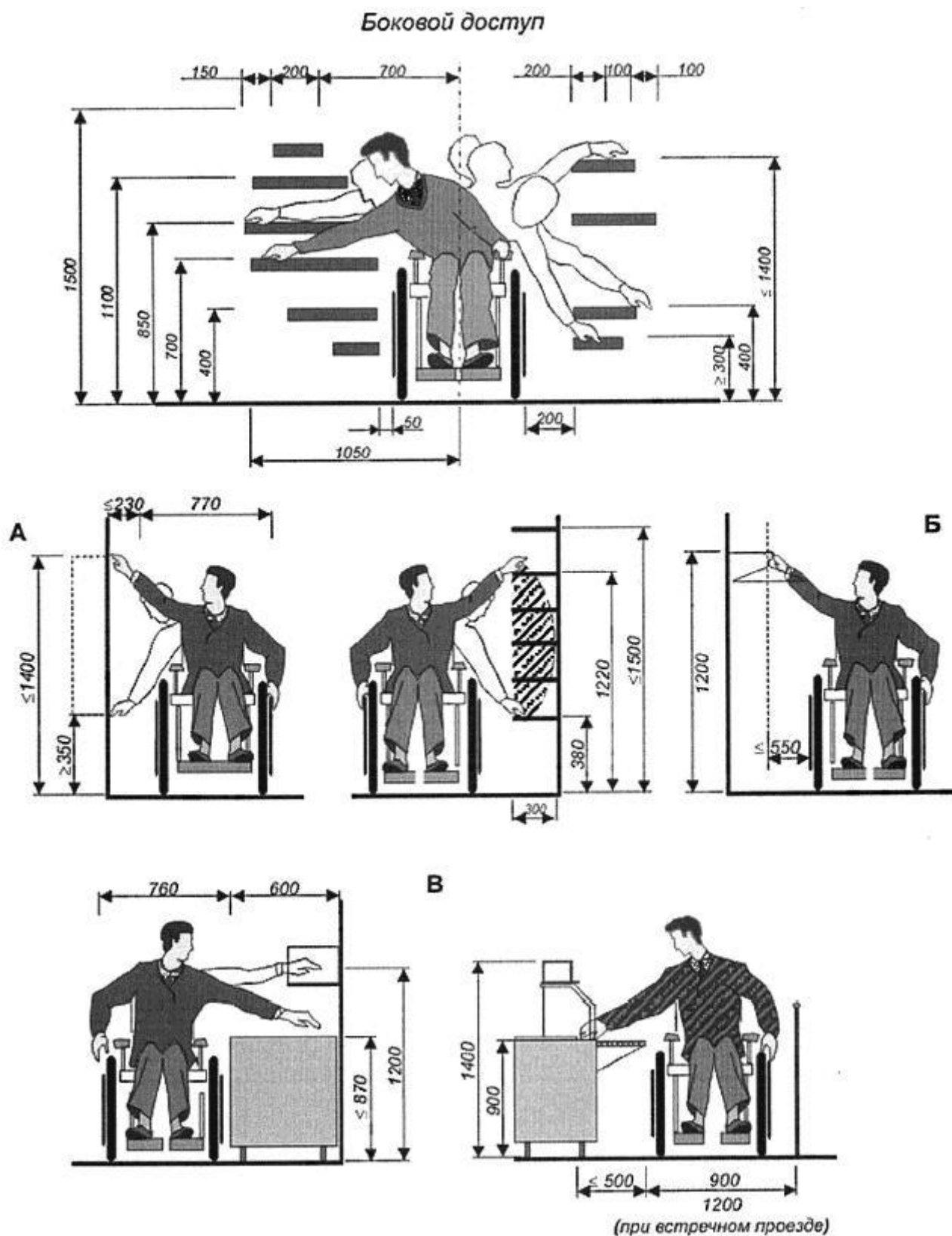
Рисунок Г.3 - Досыгаемость
