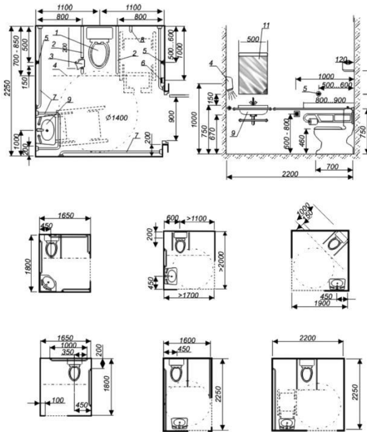
Рисунок Г.7 - Примеры оборудования кабин общественных уборных
